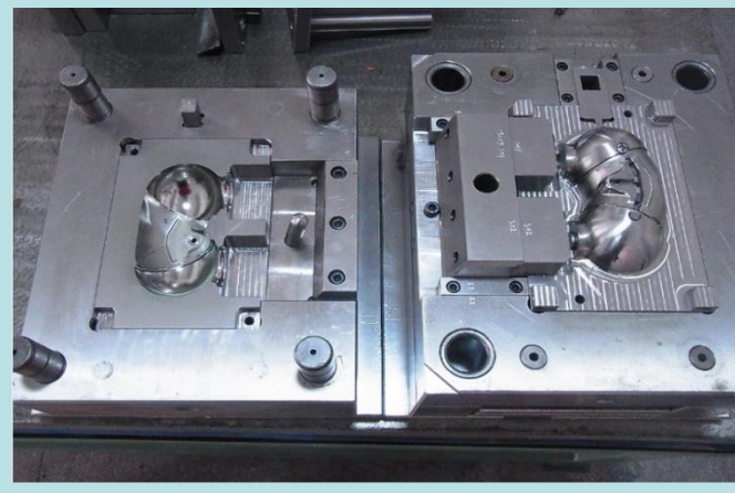
側抽芯結構
