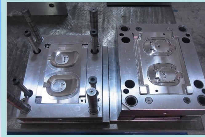
三板模細水口
