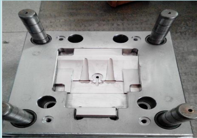
圓弧抽芯結構
